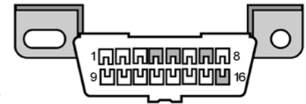
рис.12 Контакты колодки ОБД2
