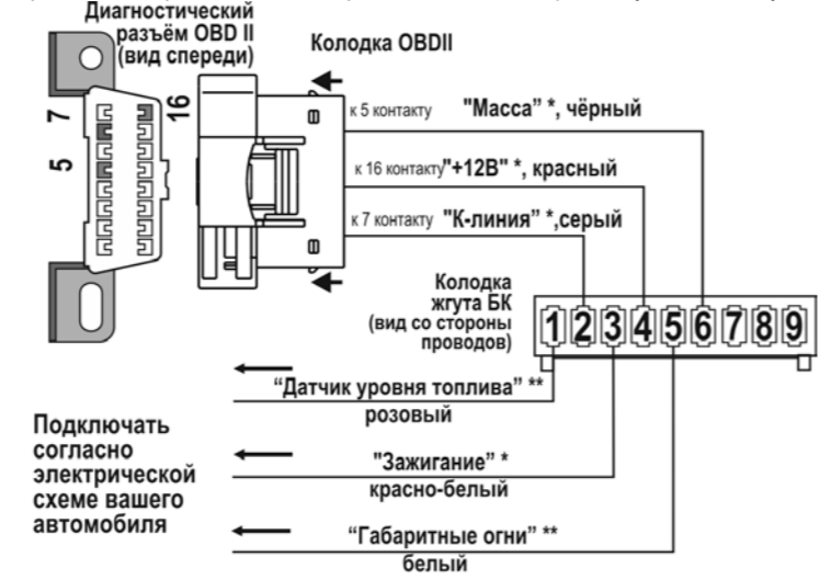
* Подключать обязательно ** Опциональное подключение рис.15 Схема подключения к а/м семества ЗАЗ.
