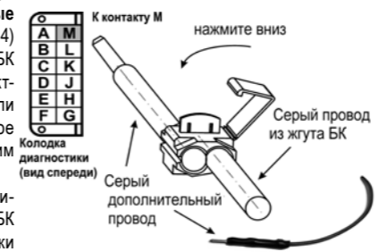
рис.20 Схема подключения дополнительного сигнализации. При помощи зажимов провода М-линии
