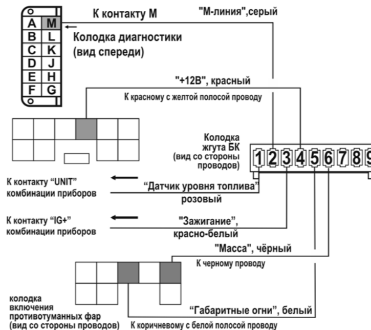
рис.11 Схема подключения к а/м ЗАЗ Ланос Т150 (ЕВРО-2)
