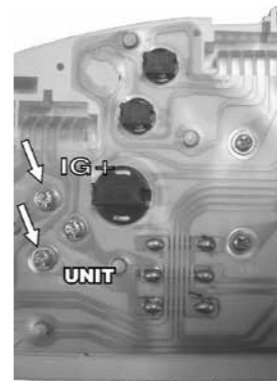
рис.9 Печатная плата комбинации приборов
