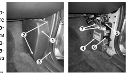
рис.17 контроллер ЭСУД Daewoo Nexia
