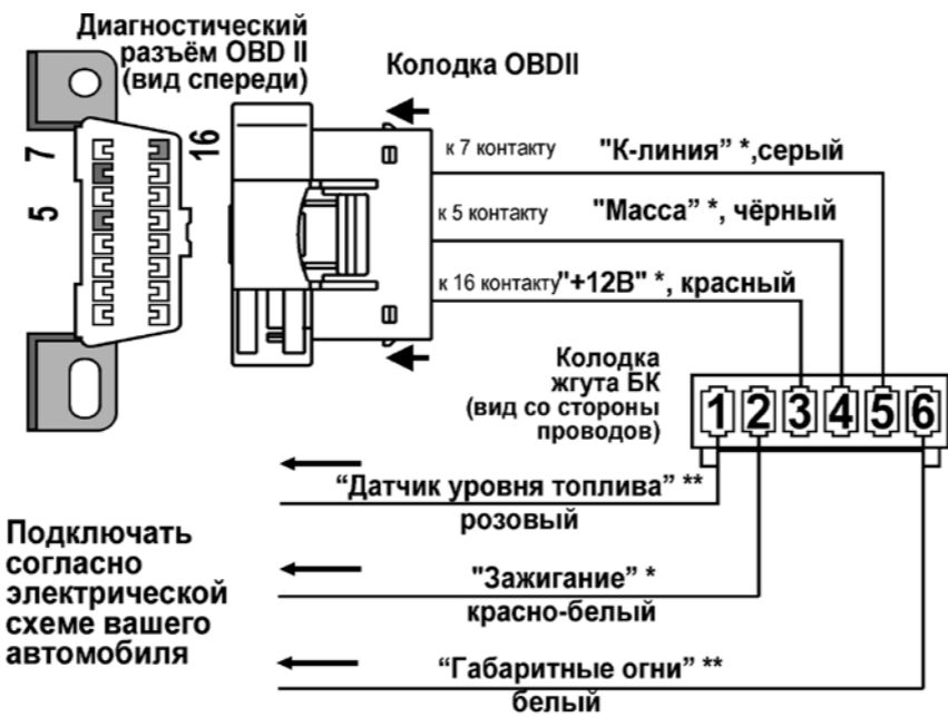
рис.15 Схема подключения к а/м Chevrolet Lacetti и Aveo.
