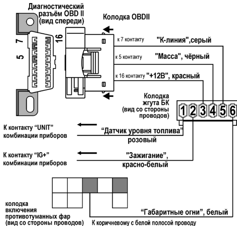
рис.14 Схема подключения к а/м Chevrolet Lanos (после 2008 г.в.) (EBPO-3)
