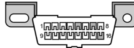
рис.12 Контакты колодки ОБД2
