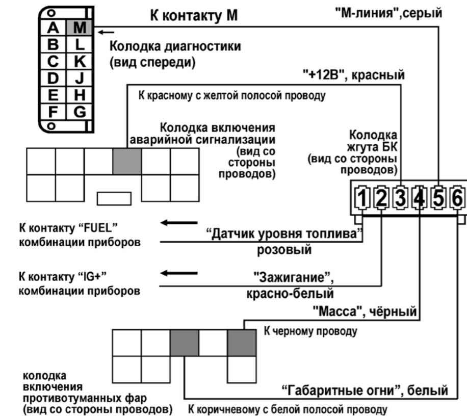
рис.13 Схема подключения к а/м Daewoo Nexia (до 2008 г.в.) (EBPO-2)
