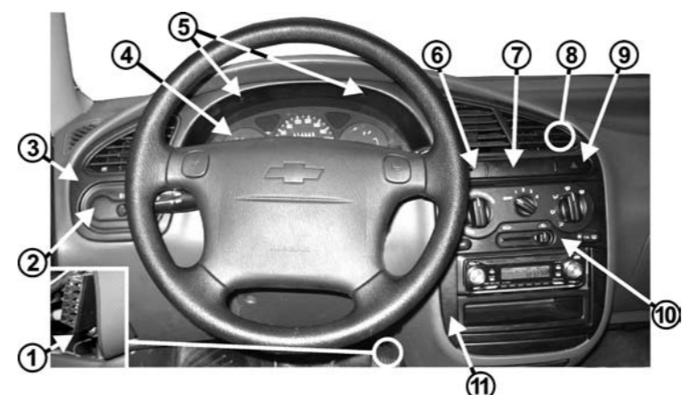
рис.8 Панель приборов а/м Chevrolet Lanos
