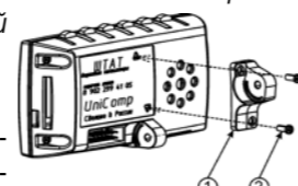
рис.16 Крепление кронштейна к корпусу БК
