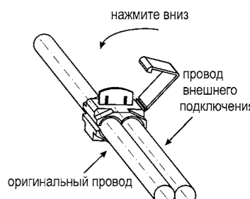
рис.10 Соединение проводов через зажим
