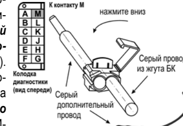
рис.11 Схема подключения диагностики согласно схеме подключения дополнительного провода М-линии
